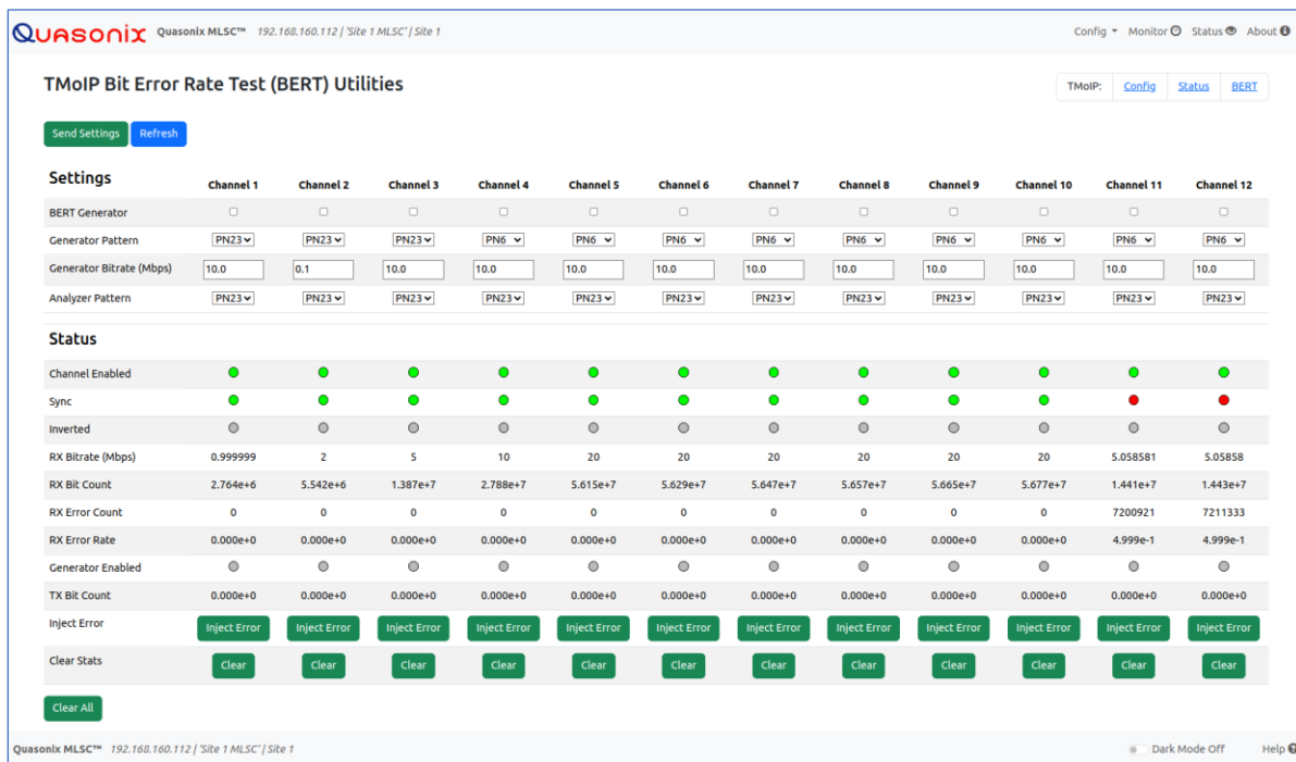
Figure 43: Bit Error Rate Test (BERT) Utilities
